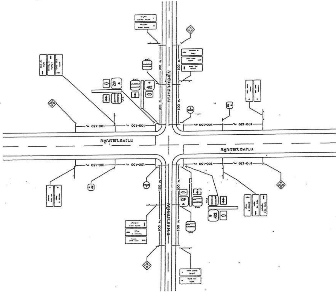
แสดงการติดตั้งป้ายหมายเลขทางหลวงท้องถิ่น (ถนน-1/1) บริเวณสี่แยก ( เชื่อมทางหลวงแผ่นดิน )
