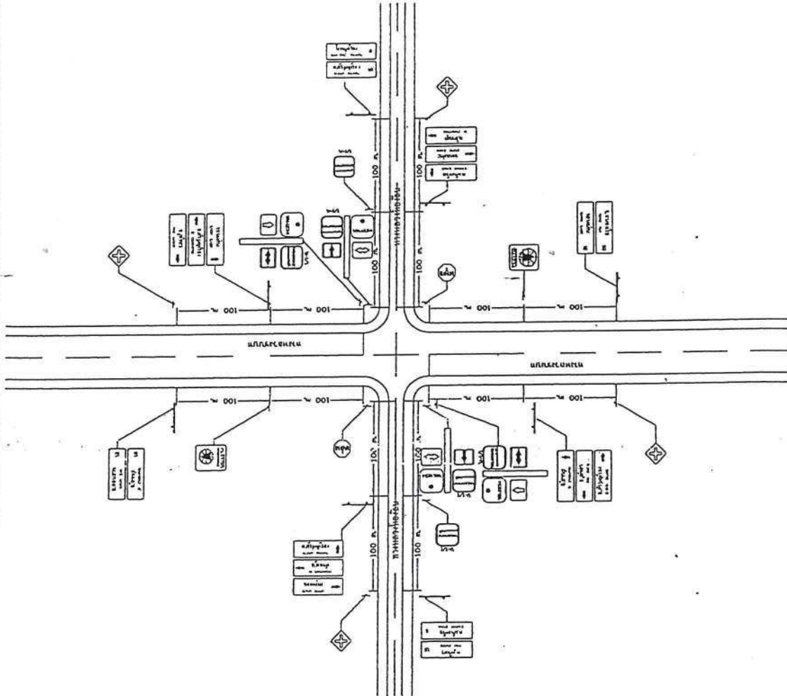
แสดงการติดตั้งป้ายหมายเลขทางหลวงท้องถิ่น-1/บริเวณสี่แยก ( กรณีเชื่อมทางหลวงชนบท )
