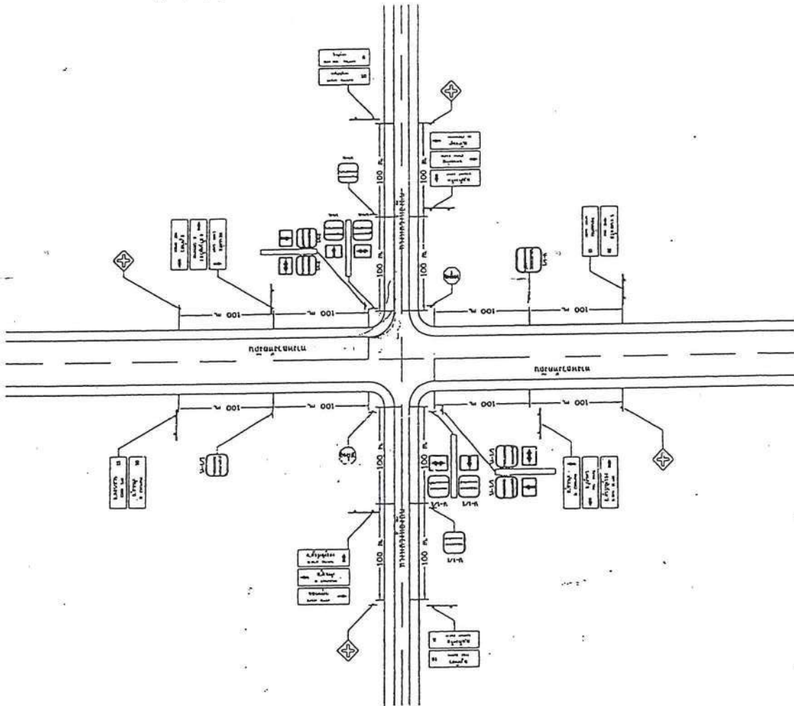
แสดงการติดตั้งป้ายหมายเลขทางหลวงท้องถิ่นแบบ-1/1บริเวณสี่แยก ( กรณีเชื่อมทางหลวงท้องถิ่น )
